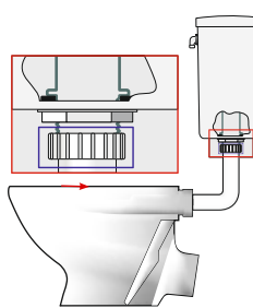
Siphon Cap Nut
